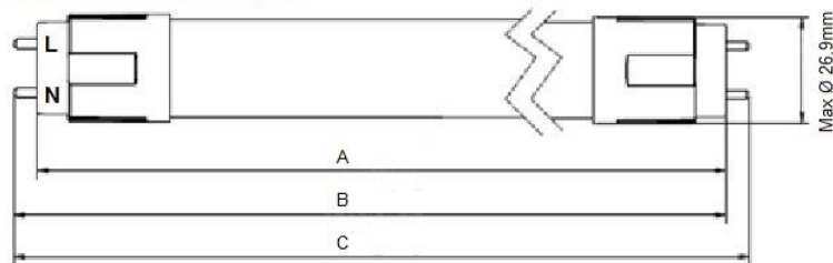
Figura 3 – utilizzo con apparecchio d'illuminazione con reattore, senza apportare modifiche
